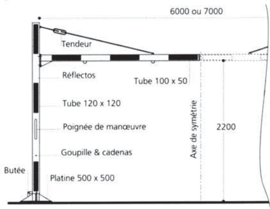
Portique tournant avec tirants
