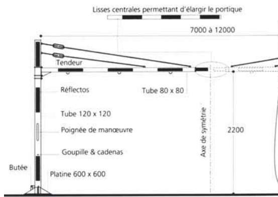
Portique tournant universel avec tirants
